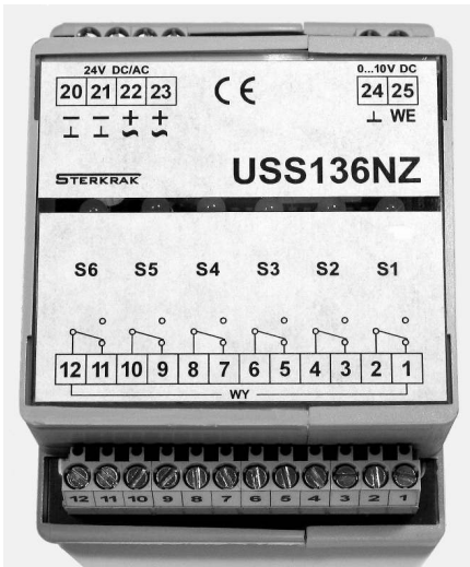
Fig.1 The USS136NZ module.
