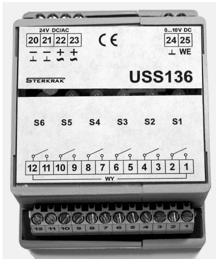
Fig.1 The USS136 module.
